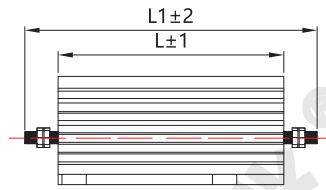
图一 (主视图)
