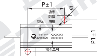
图三 (俯视图)
