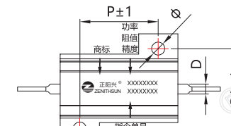
图三 (俯视图)
