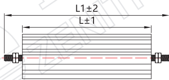
图一 (主视图)
