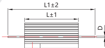
图一 (主视图)
